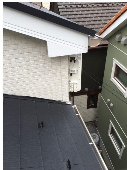
横浜市神奈川区新小安 壁面取付 デザインアンテナ工事
