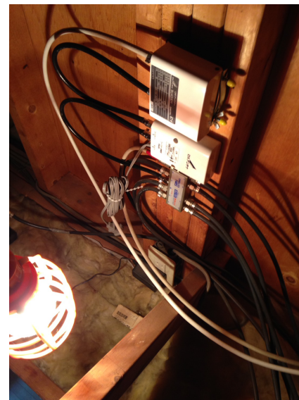
横浜市神奈川区羽沢南 6 分配器 ブースター本体 ブースター電源部
