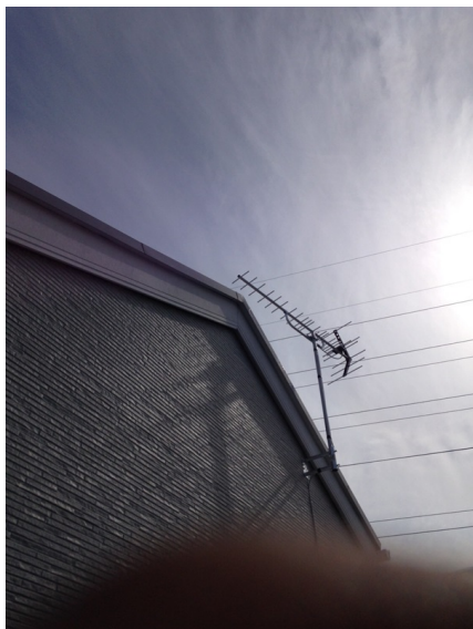
横浜市港北区高田西 壁面取付 地デジアンテナ 工事
