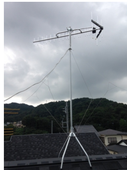
秦野市渋沢上 垂直偏波受信 地デジアンテナ屋根上工事
