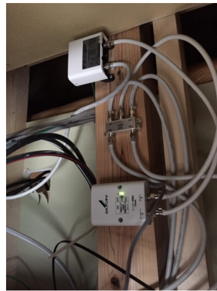
茅ヶ崎市矢畑 ハートフルホーム様物件 ブースター電源部 ブースター本体 4分配器
