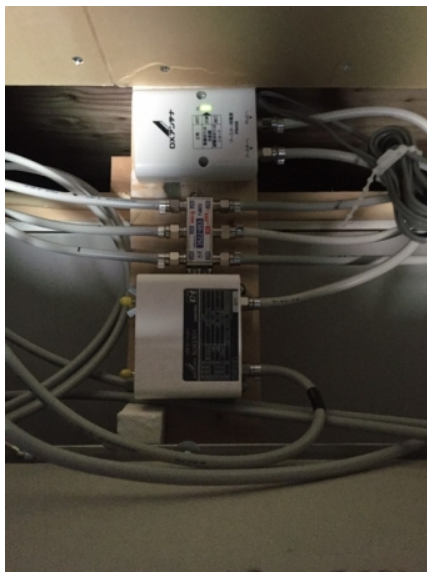
茅ヶ崎市平和町 ディーハウス様物件 ブースター電源部 ブースター本体 5分配器
