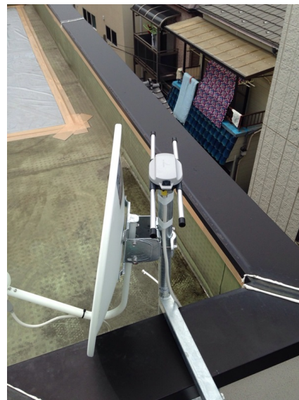
品川区西中延 リアルトハーツ様物件 デザインアンテナ工事後の外観
