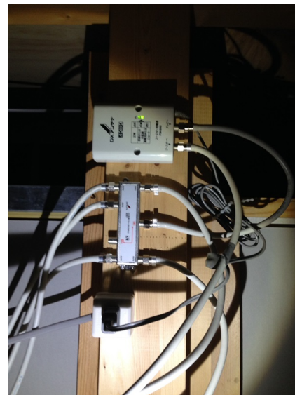
足立区興野 壁面取付 デザインアンテナ工事
