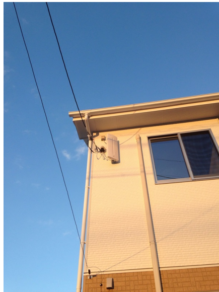
久喜市南栗橋 セルコホーム様物件 地デジアンテナ屋根上工事
