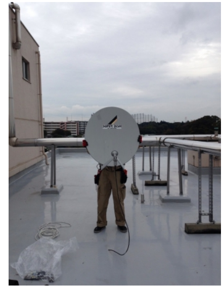
川口市安行領根岸 集合住宅用BSアンテナ
