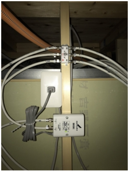
川口市戸塚南 ブースター電源部 5分配器
