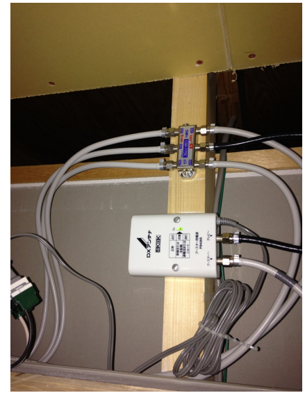
川口市戸塚南 5分配器 ブースター電源部
