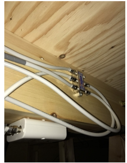
川口市青木 ブースター電源部 5分配器
