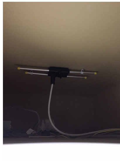
市川市原木 三栄建築設計様物件 地デジアンテナ屋根裏工事
