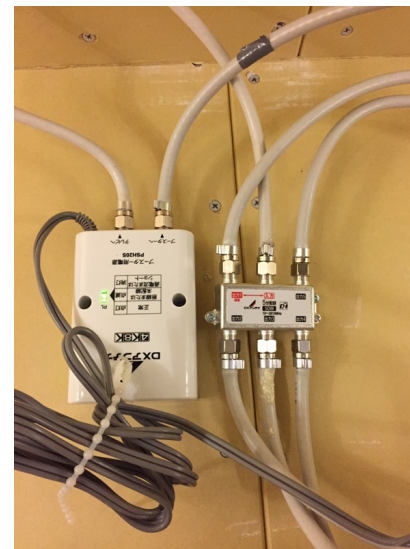
市川市鬼高 三栄建築設計様物件 ブースター電源部 5分配器
