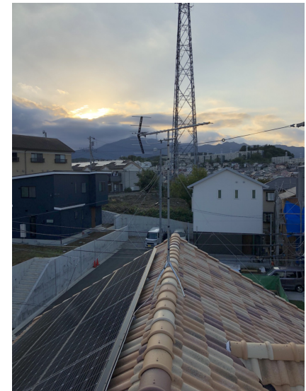
厚木市温水西 屋根上設置 八木式アンテナ工事
